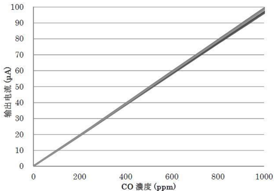
图 2: NE-CO-BL 气体感应度
