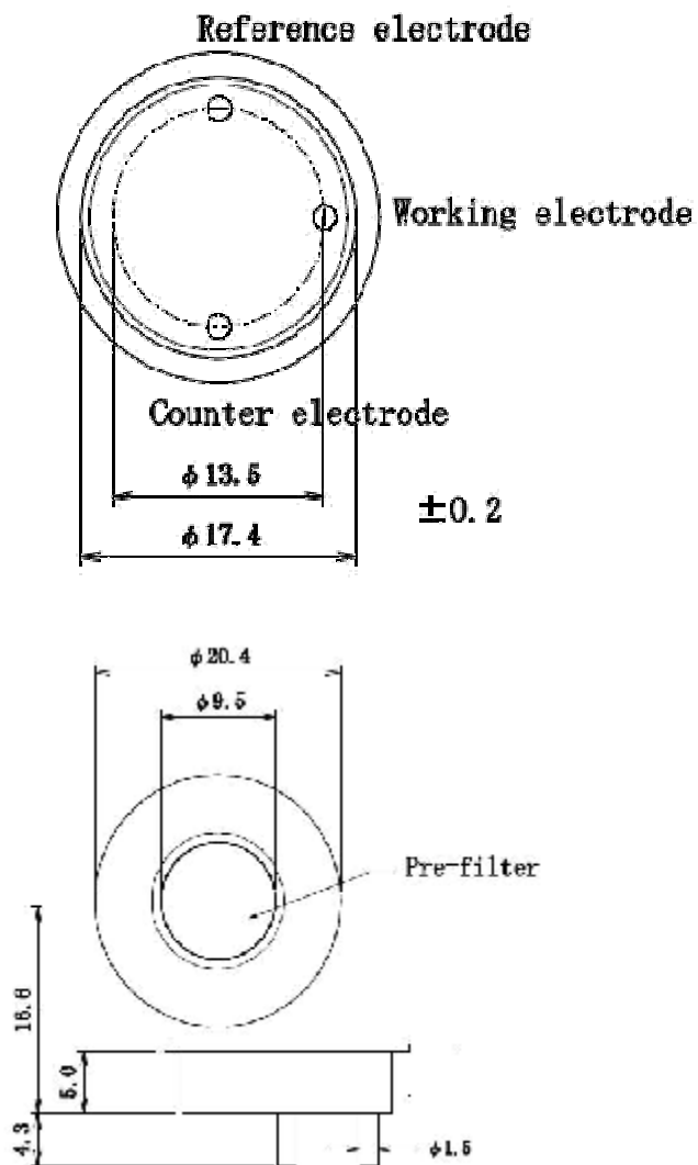
图 1: 外观 尺寸
