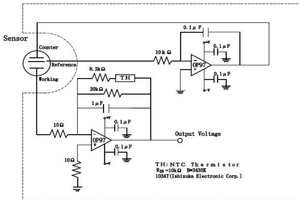
图 4: 推荐测试电路
